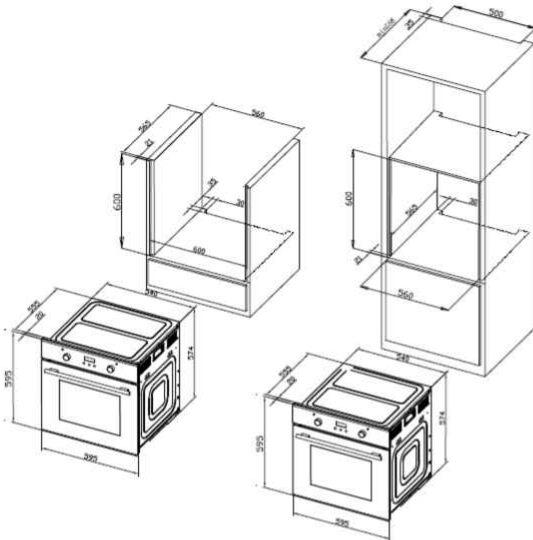
Einbauweise 1
